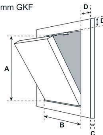
Krídlo dveriek je vyberateľné
