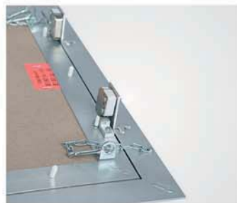
Vyvesiteľné krídlo dvierok
